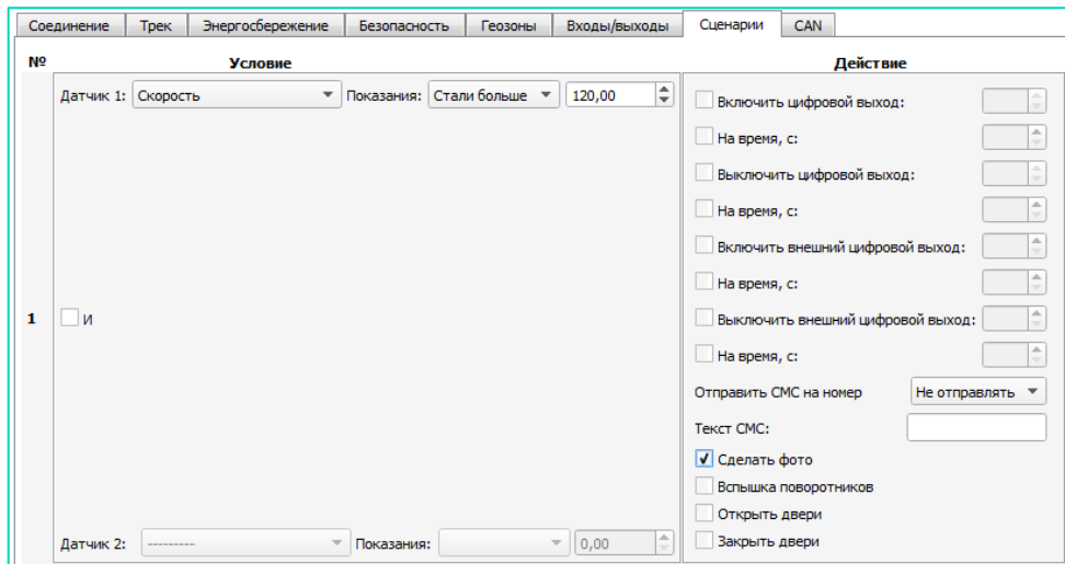
Рис. 5.10. Сценарий создания фотоснимка при скорости более 120 км/ч
