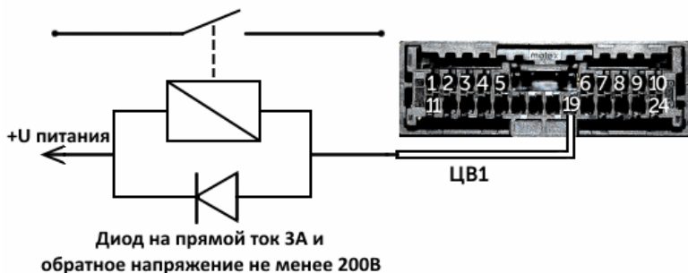
Рис. 4.6. Схема подключения реле на Цифровой выход 1.
