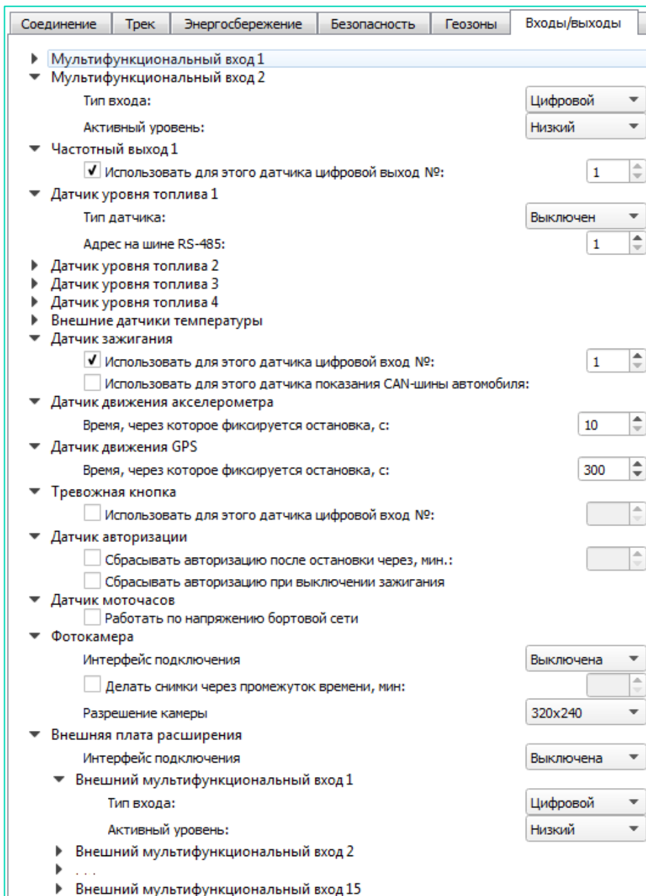
Рис. 5.9. Настройки вкладки «Входы/выходы».
