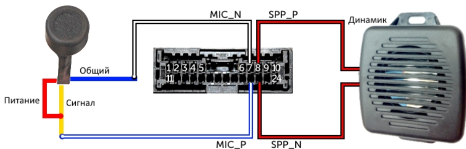
Рис. 4.7. Схема подключения микрофона и динамика.
