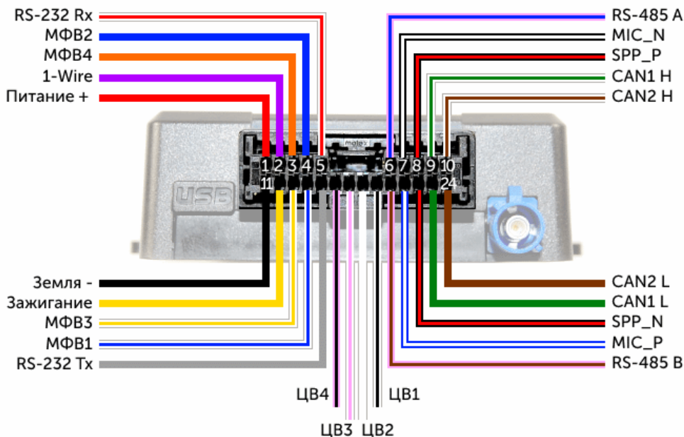
Рис. 3.1. Расположение контактов в разъёме.
