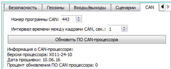
Рис. 5.11. Настройки для CAN-сервиса.
