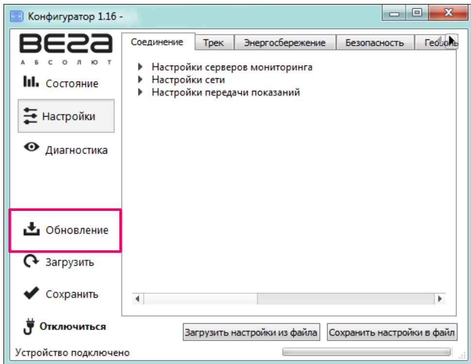
Рис. 5.13. Кнопка «Обновление».
